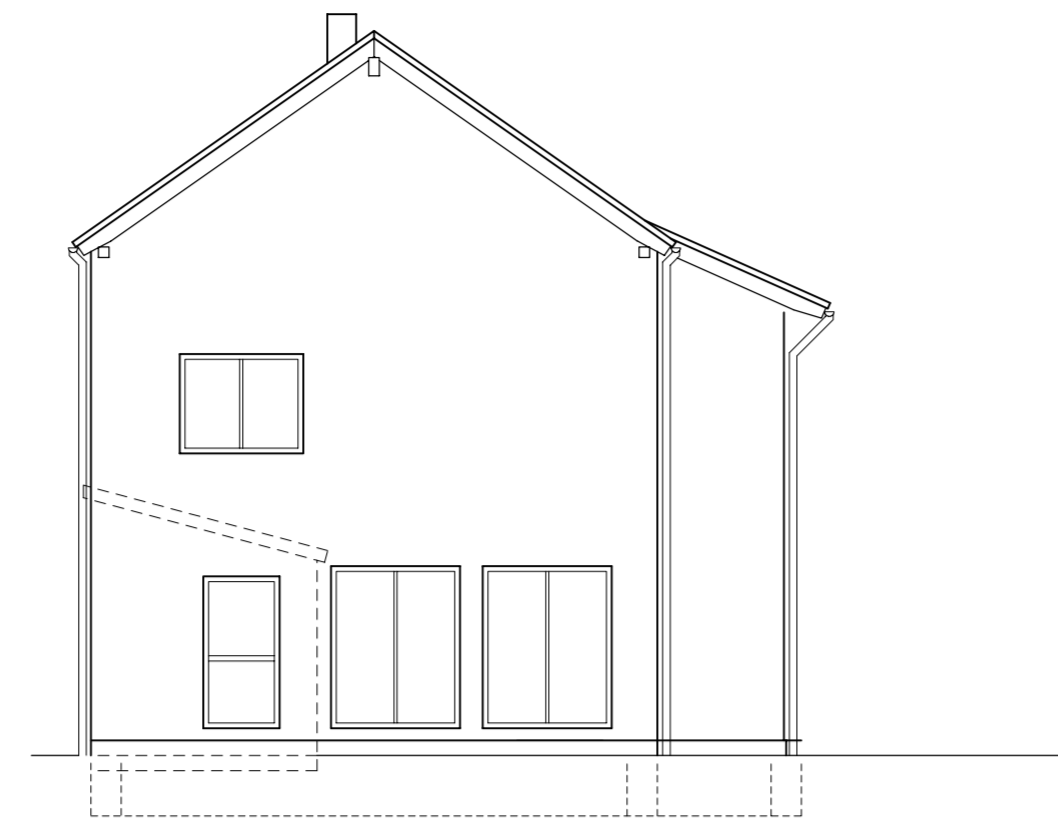
ANSICHT "West"
