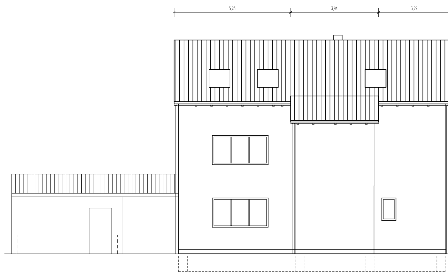
ANSICHT "Süd"
